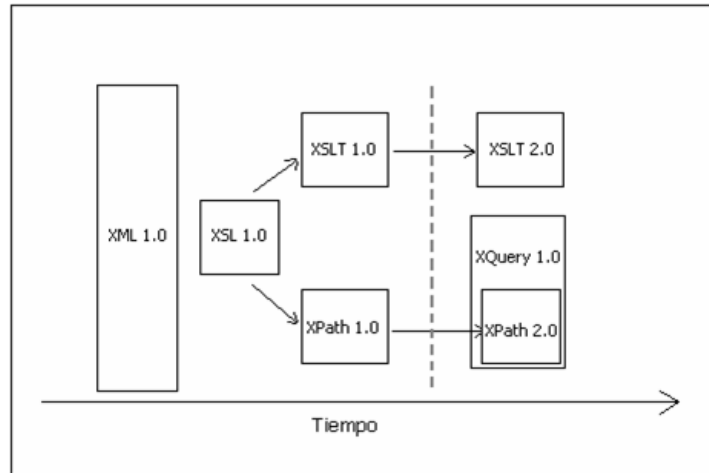
Figura 1. XQuery y su relación con los estándares W3C
